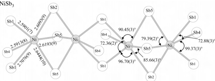
\alpha -CeNiSb 3
